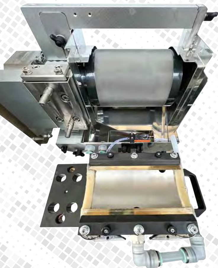
Il sistema Adaptive Ink Chamber con la camera chiusa aperta. El sistema Adaptive Ink Chamber con la cámara de rasqueta abierta.
